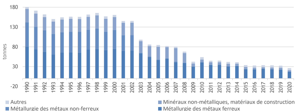
Répartition des émissions de Pb du secteur de l'industrie manufacturière et construction en France (Métropole)
