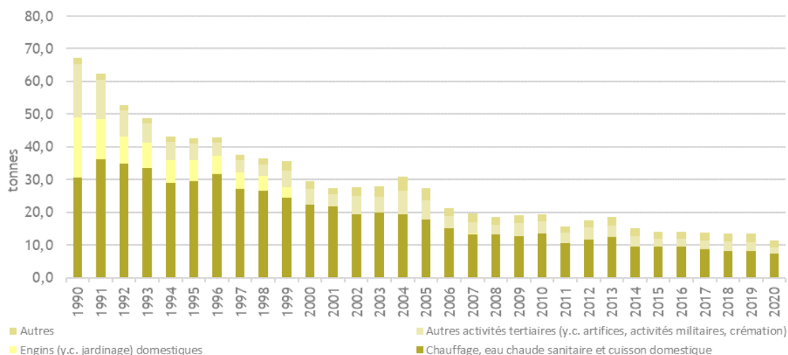
Répartition des émissions de Pb du secteur du résidentiel/tertiaire en France (Métropole)
