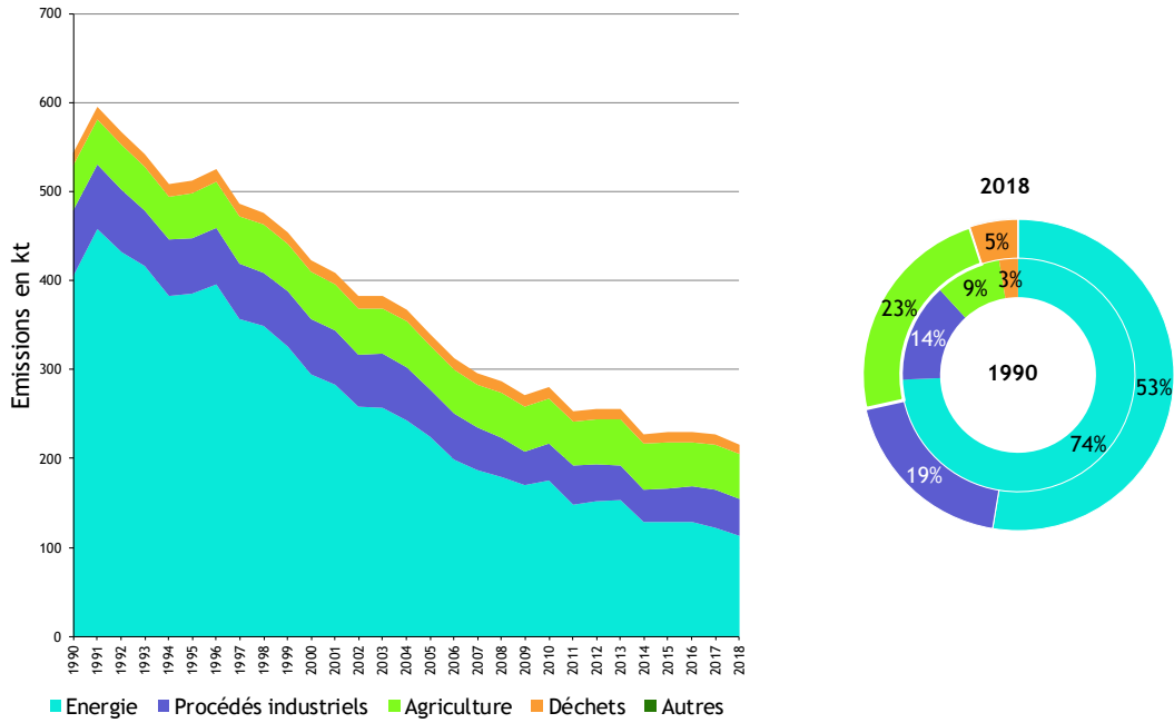
Figure 29 : Evolution et répartition des émissions de PM 10 en France métropolitaine
