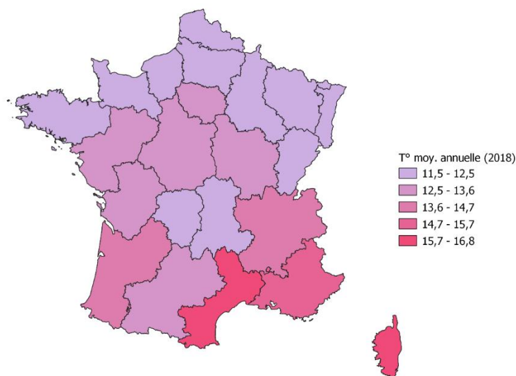
Figure 108 : Températures moyennes annuelles régionales
