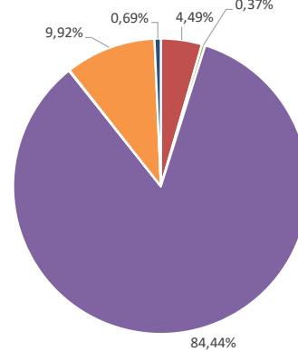
Procédés industriels - COVNM (2018)
